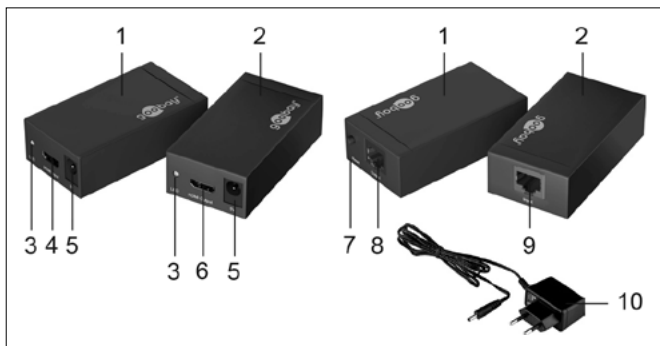
Fig.: Elementi di comando e parti di prodotto
