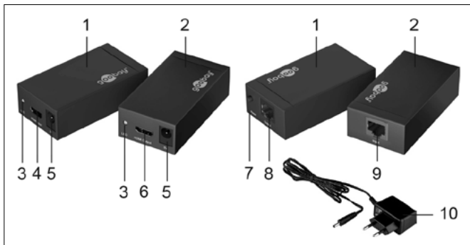
Fig.: Éléments de commande e pièces
