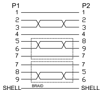
Anschlussdiagramm / Wiring diagram
